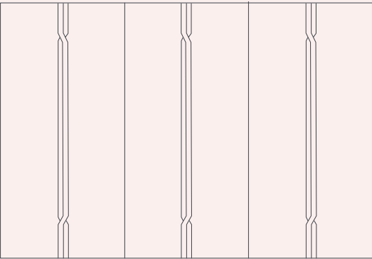
BOLASCO 6 ANTE W 354 D 66 H 258 cm
