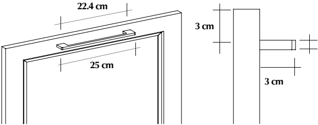
maniglia a ponte alluminio lucido, titanio o nero WZ2 bright aluminium, titanium or black bridge handle WZ2 poignée à pont aluminium brillant, titanium ou noir WZ2 Tirador en puente aluminium brillant, titanium o negro WZ2
